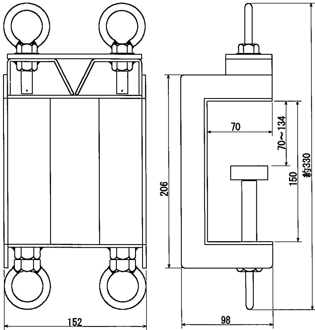
裝備金具18型外形寸法図
